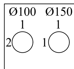
кабловска канализација у 1 реду са 4 отвора Ø100 и једним Ø150
