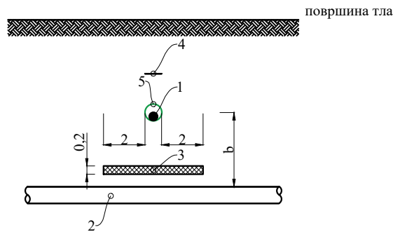
ПРЕСЕК 1-1
