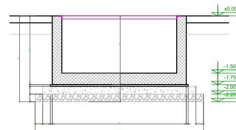
ŠAHT ELEVATORA, R=1:100
