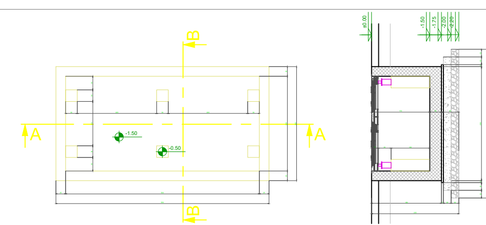
PRESEK A-A
