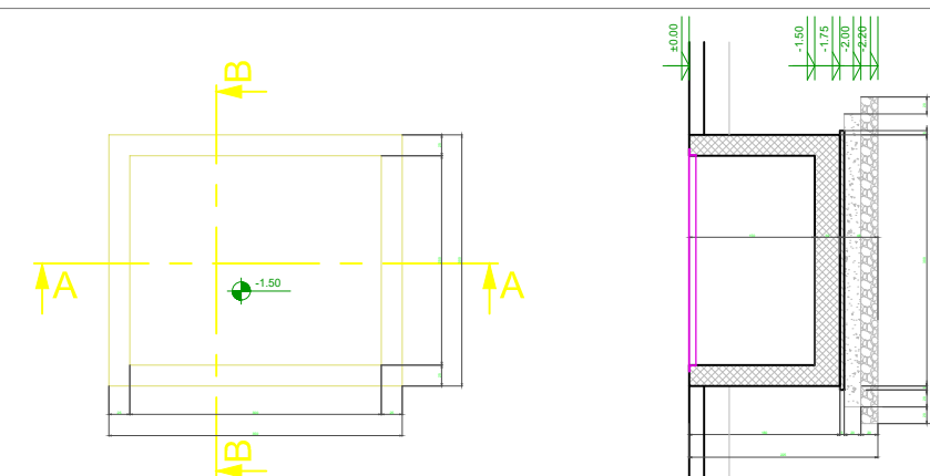
PRESEK A-A
